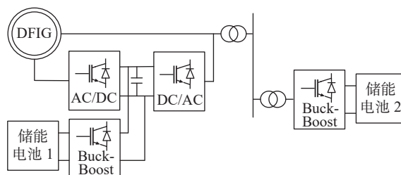
图 3 储能系统接入位置示意图
