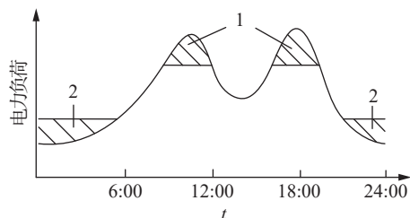
图 2 削峰填谷示意图
