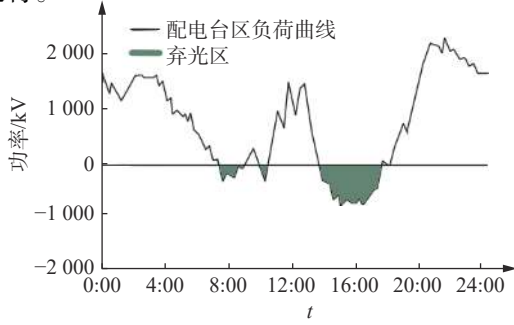
图4 分布式能源消纳示意图
