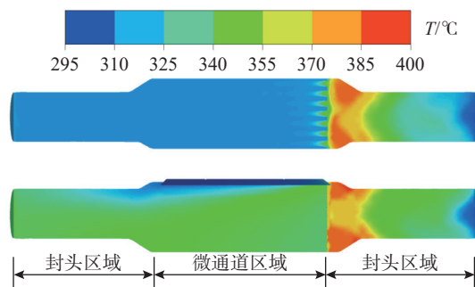
图 3 反应器内温度分布云图
