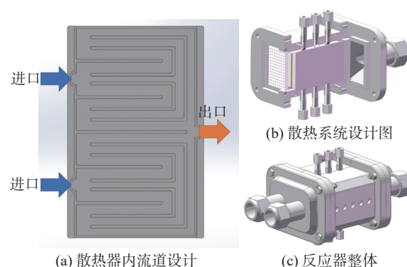
图 6 反应器设计
