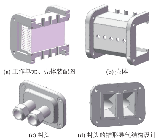
图 5 反应器设计
