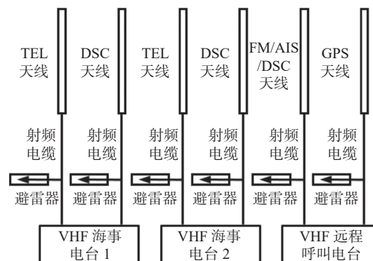
图5 VHF 对船通信系统结构图
