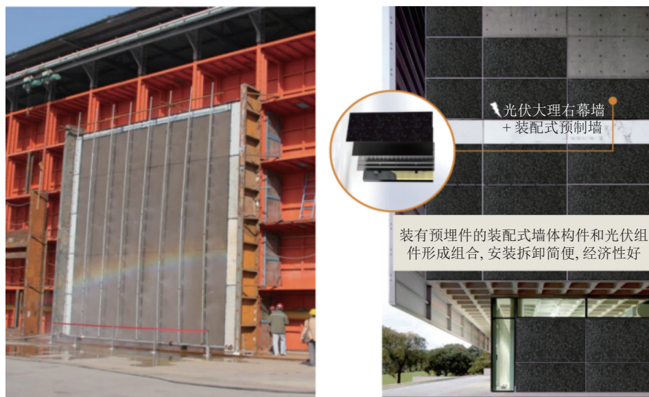
图6 装有预埋件的装配式墙体构件和光伏大理石组件形成组合
