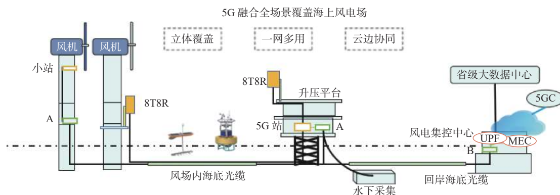
图 9 5G 融合 STN 立体网络覆盖
