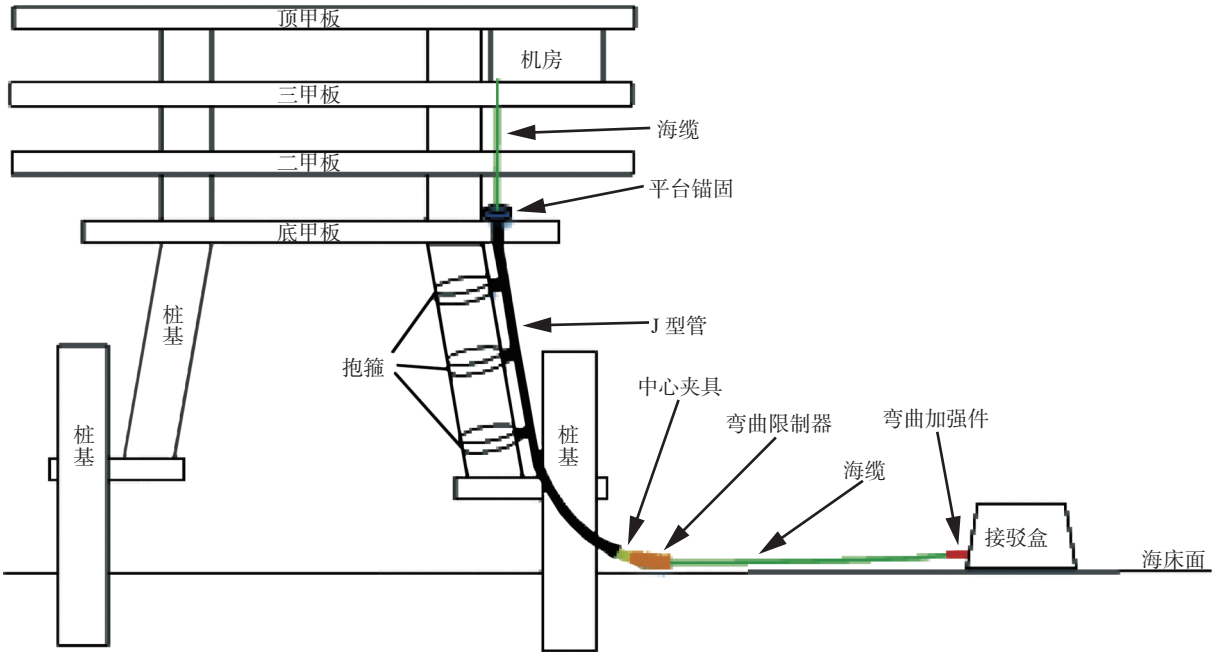
图 8 水下光网通信 Fig. 8 Underwater optical network communication
