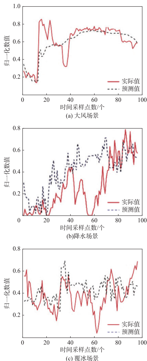
图 3 吉林某风电场转折性天气过程下风电功率预测偏差 [48]
