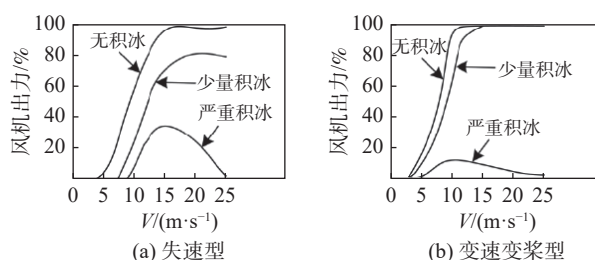
图2 积冰对不同控制方式风机出力的影响 [57]
