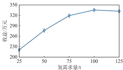
图 10 氢需求量对氢能电站经济性的影响
