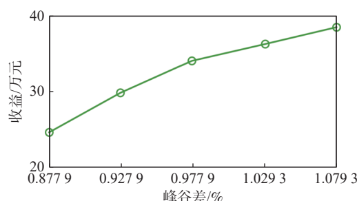
图 7 电价峰谷差对氢能电站经济性的影响
