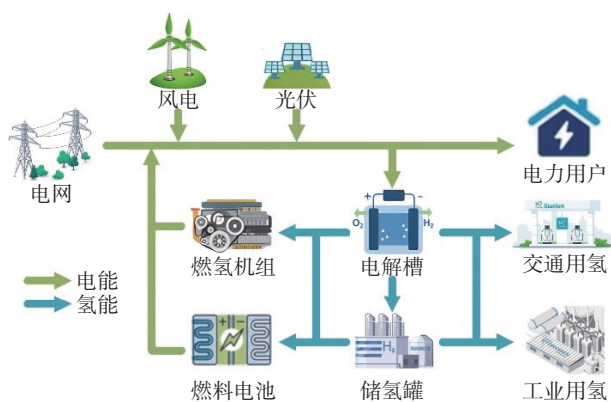
图 1 电-氢互补协同系统结构
