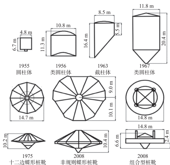
图 2 不同桩靴形式 [5]
