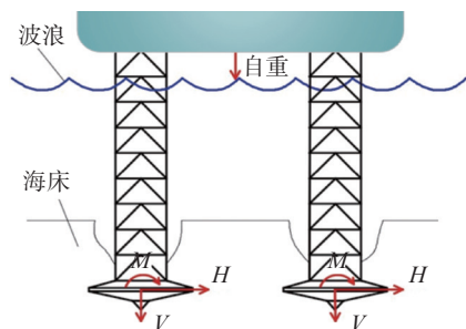
图 4 桩靴基础受力情况
