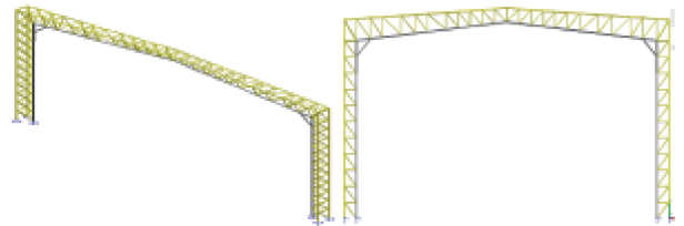
图5 户内直流场典型横向受力体系
