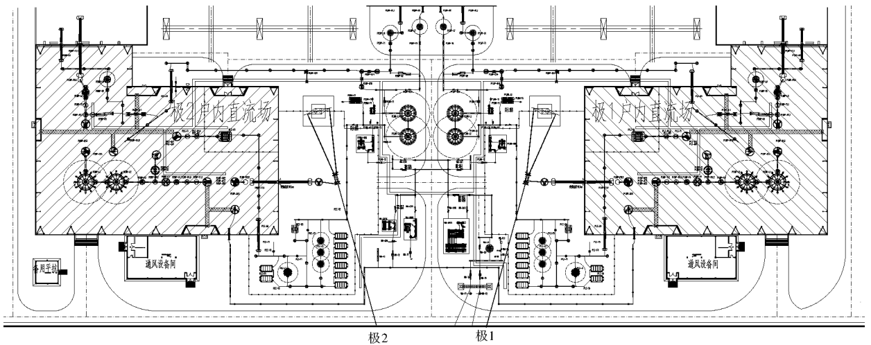
图1 户内直流场在换流站内平面位置示意图
