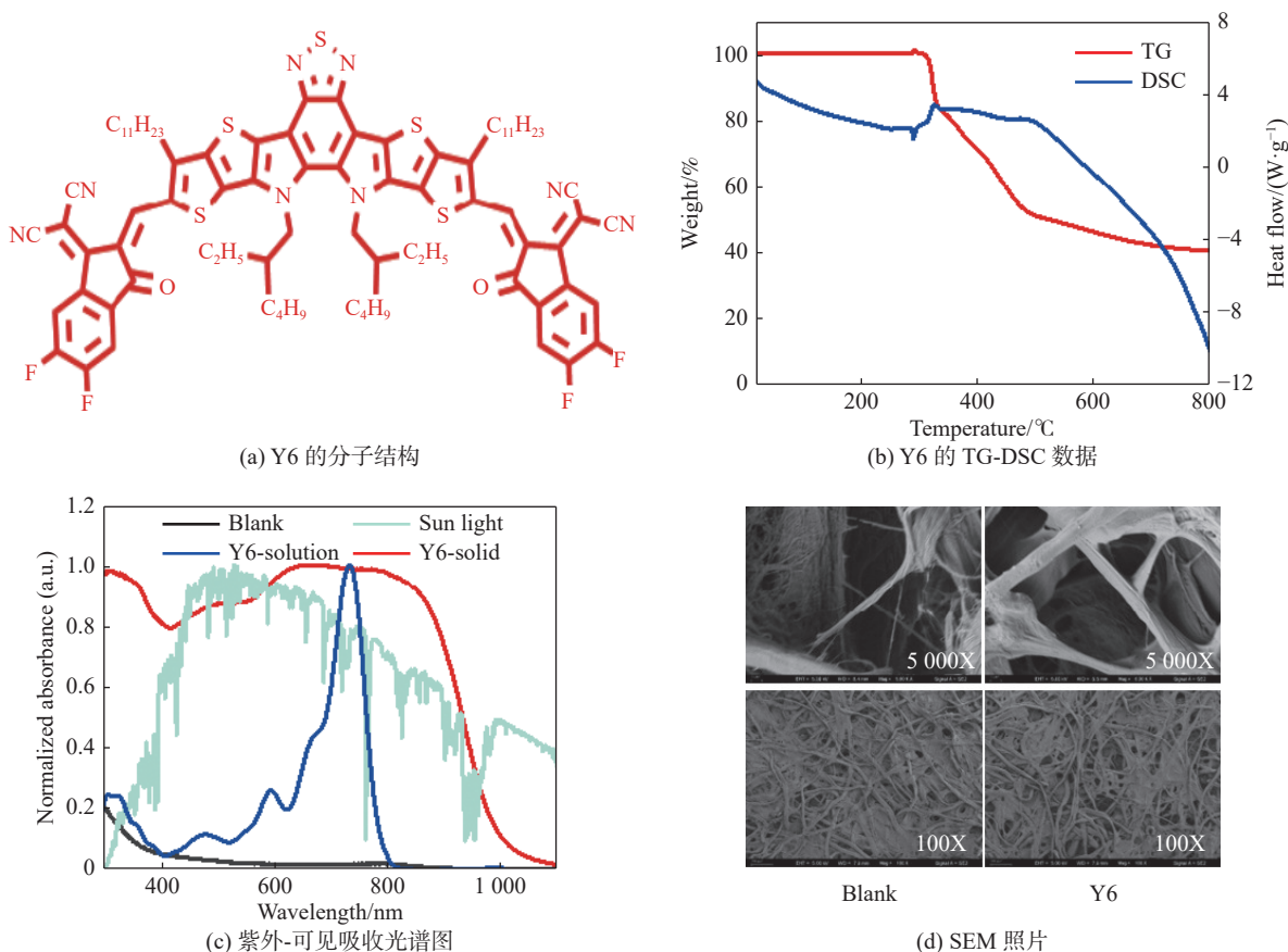
图 2 材料表征
