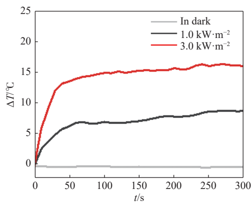
(b) 不同光强下集成热电器件表面与水的温差图
