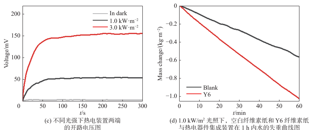
图5 水电联产性能
